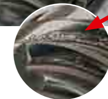
Hier sind kleine Ausbrüche an den Zahnflanken deutlich zu erkennen.
